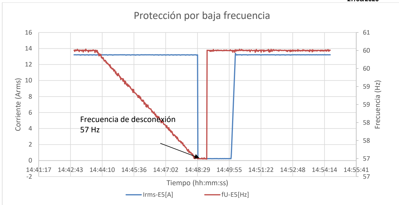
Figura 22. Disparo por Baja Frecuencia.
