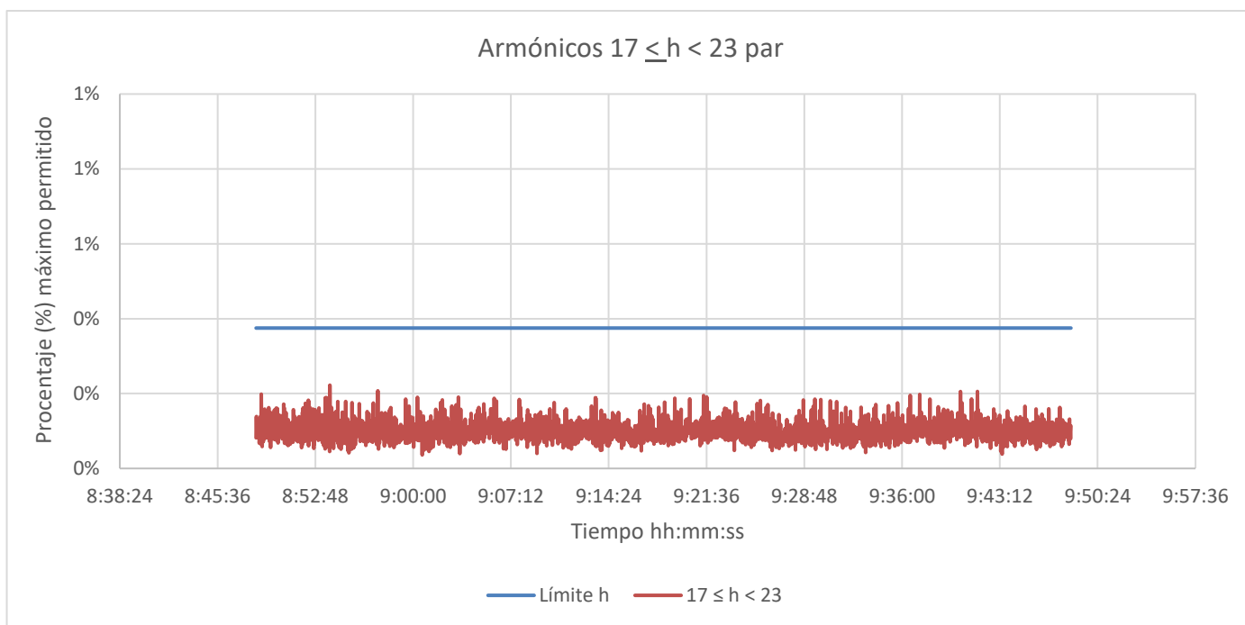
Figura 12. Armónicos 17 \leq h < 23 par.
