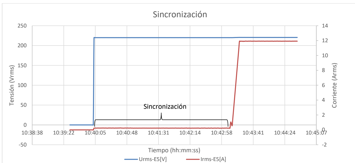
Figura 3. Gráfica de sincronización.
