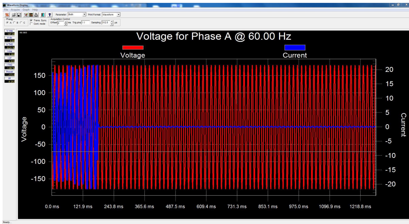
Figura 23. Tiempo de desconexión en alta frecuencia 61.2Hz
