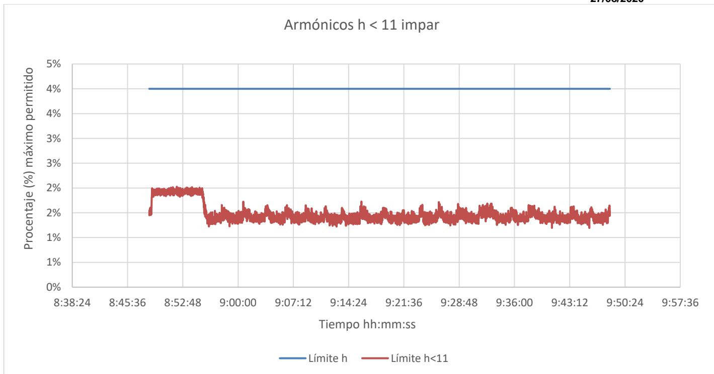
Figura 5. Armónicos h < 11 impar.
