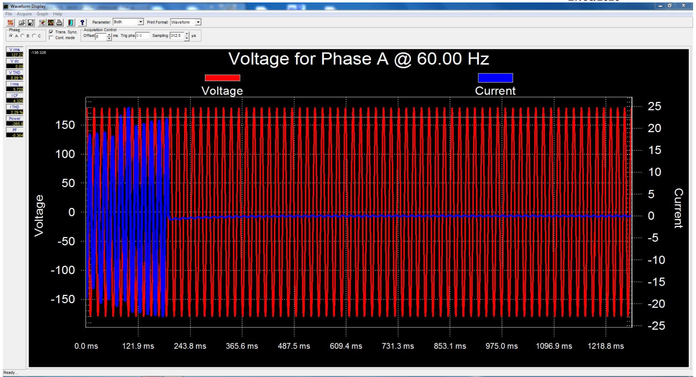
Figura 24. Tiempo de desconexión en baja frecuencia 57Hz.
