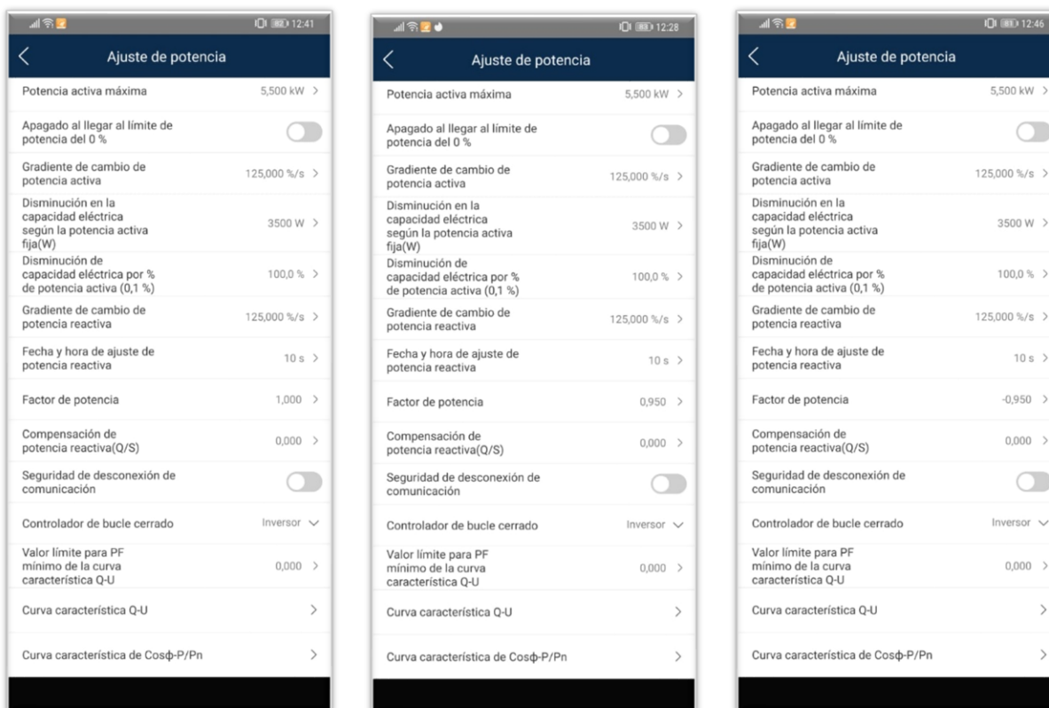
Figura 4. Configuración del factor de potencia en aplicación móvil "FusionSolar".
