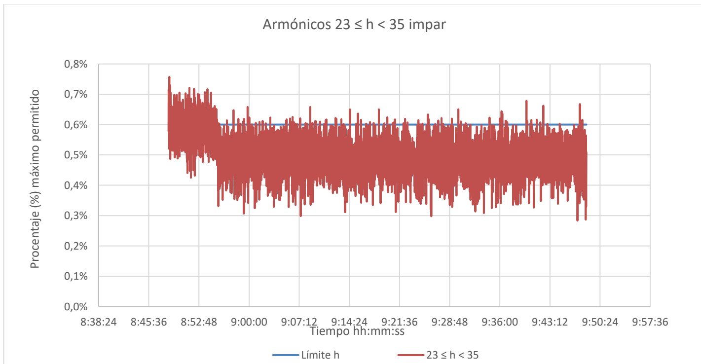
Figura 8. Armónicos 23 \leq h < 35 impar
