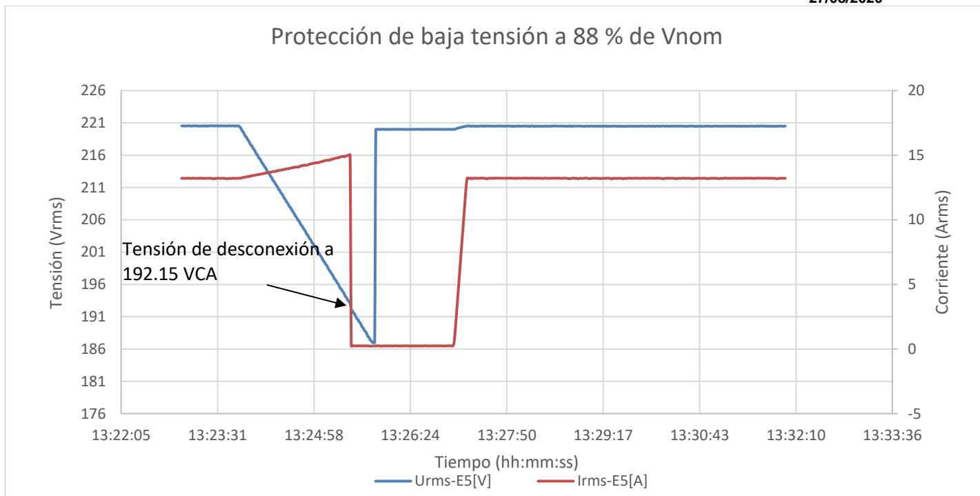
Figura 15. Desconexión por baja tensión.
