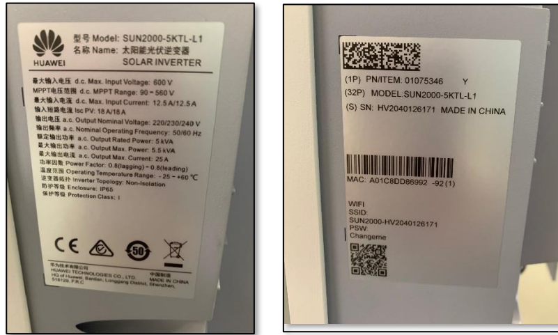
Fotografía 1. Fotografías y datos de placa del inversor.
