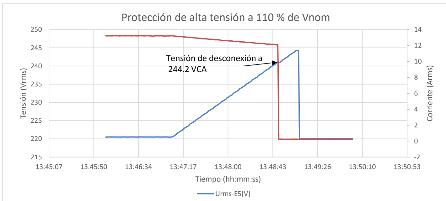
Figura 16. Desconexión por sobre tensión.
