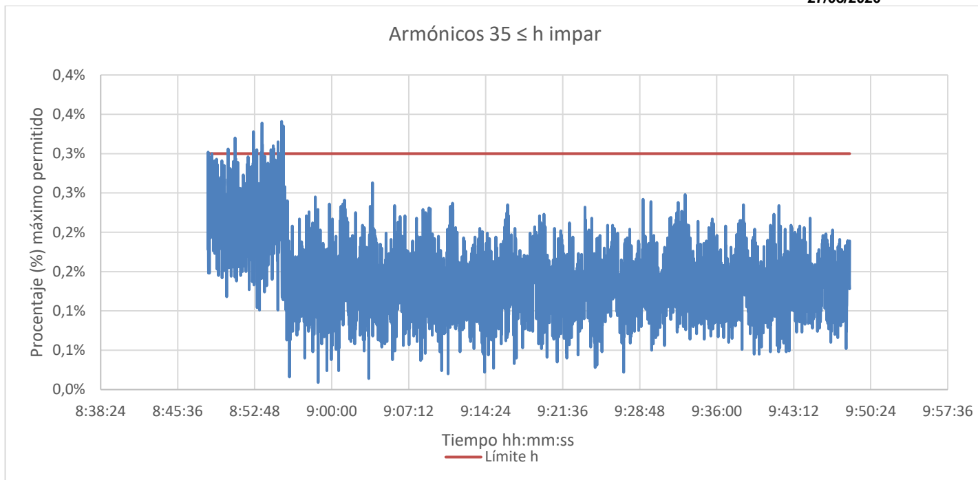
Figura 9. Armónicos 35 \leq h impar.
