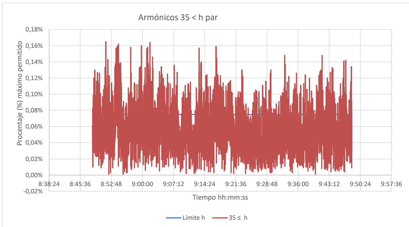
Figura 14. Armónicos 35 \leq h par.
