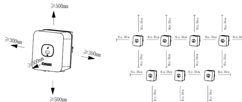
Dimensiones de espacio de un inversor Dimensiones de espacio de inversores en serie
